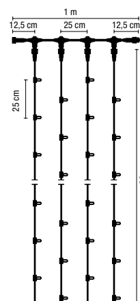
max. 4 Vorhänge koppelbar
