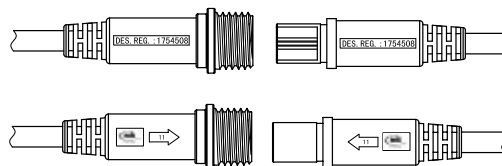
QuickFix® Verbinder – 36 Volt – 1754508
