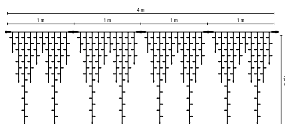
1 Kette = 4 Segmente à 1.0 m, max. 10 Ketten koppelbar
